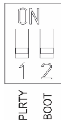
Dip-переключатели
