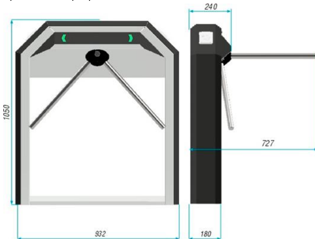
Рисунок 5.1 - Габаритные размеры турникета с планками «ТТМ-01»
