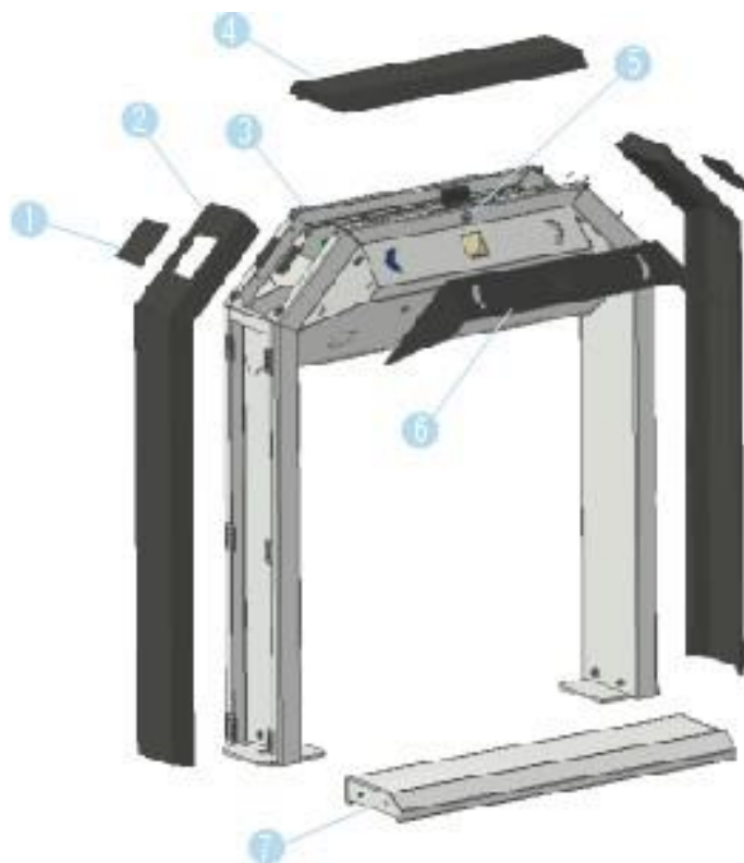
Рис. 6.1.1 - Элементы корпуса турникета «ТТМ-01»
