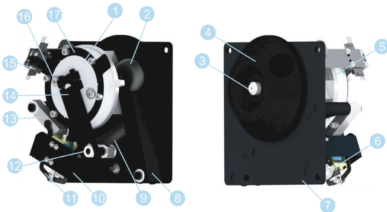
Рисунок 12.2.1 - Расположение узлов механизма турникета АТ-010
